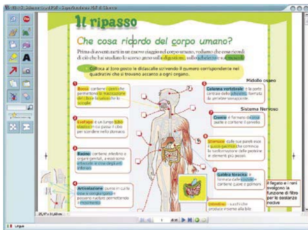
fig.3 - SuperQuaderno PDF
